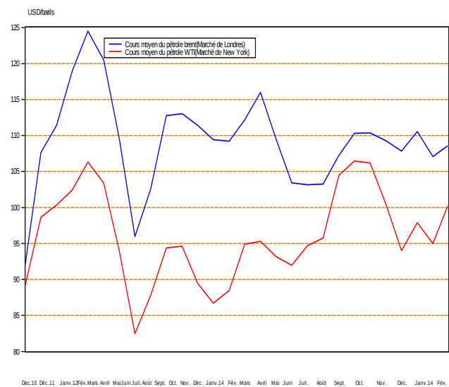
Graphique III.10 Évolution mensuelle du cours du pétrole
