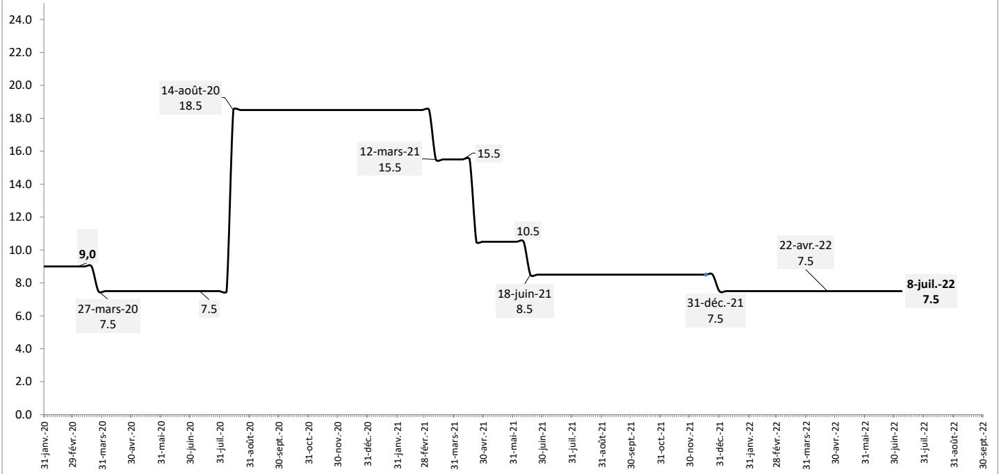
Graphique V.3. ÉVOLUTION DU TAUX DIRECTEUR AU 08 JUILLET 2022 (En %)
