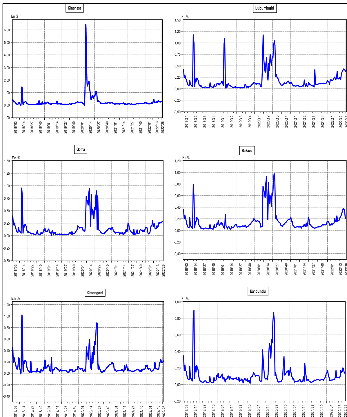
Graphique I.3 Evolution comparée de l'inflation dans les six entités provinciales de la première phase du projet IPCN 1 .
