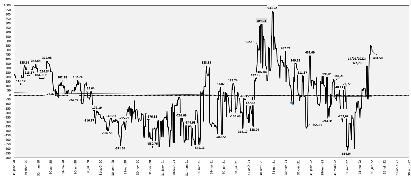
Graphique V.1. ÉVOLUTION DES AVOIRS EXCÉDENTAIRES DES BANQUES AU 01 JUILLET 2022 (En milliards de CDF)
