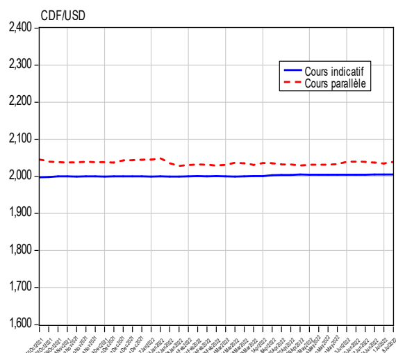
Graphique IV.1 Évolution des cours indicatif et parallèle
