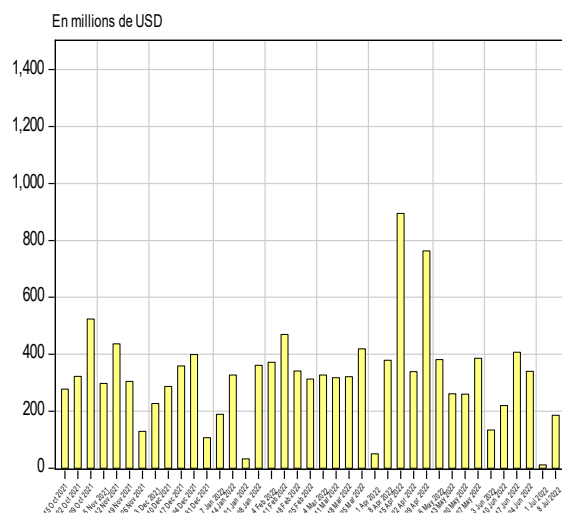
Graphique IV.4 Évolution du volume des transactions sur le marché des changes
