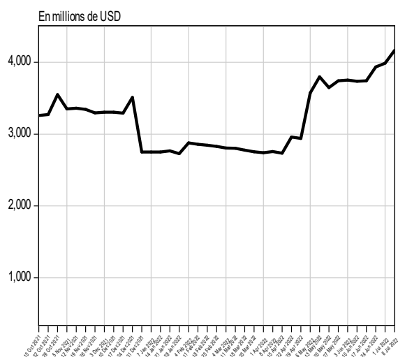
Graphique IV.6 Évolution des réserves internationales
