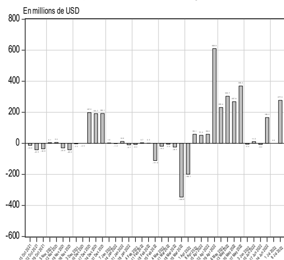
Graphique IV.5 Evolution du solde budgétaire en devises
