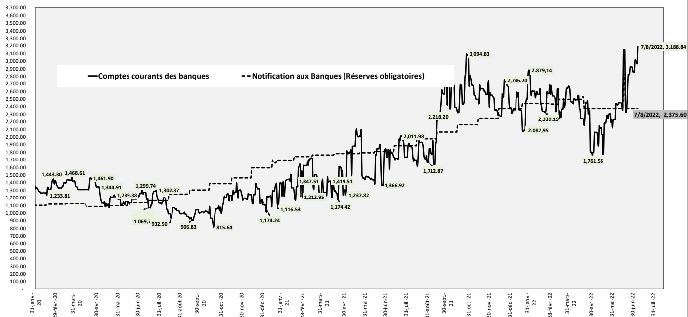
Graphique V.2. ÉVOLUTION DES COMPTES COURANTS DES BANQUES ET DES NIVEAUX NOTIFIÉS AU 08 JUILLET 2022 (En milliards de CDF)
