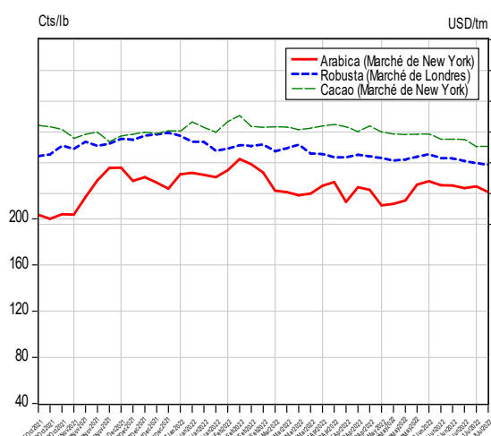
Graphique IV.11 Évolution des cours du café et du cacao sur le marché international
