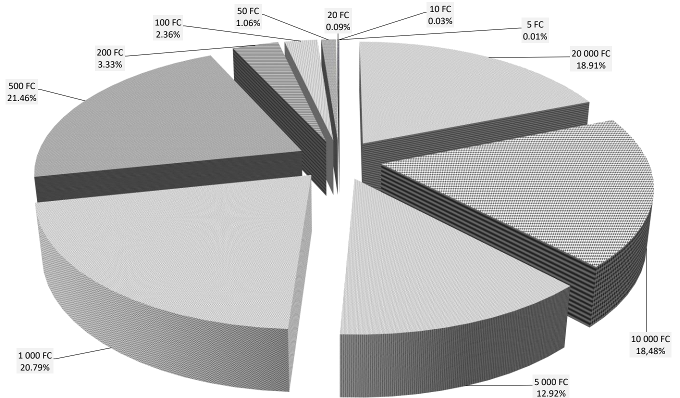
Graphique V.4. STRUCTURE DES ÉMISSIONS MONÉTAIRES PAR COUPURE AU 08 JUILLET 2022 (En % du total)
